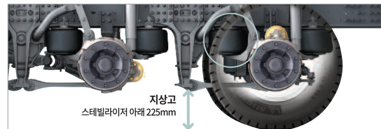
액슬 위에 장착된 에어벨로우즈/스테빌라이저바
