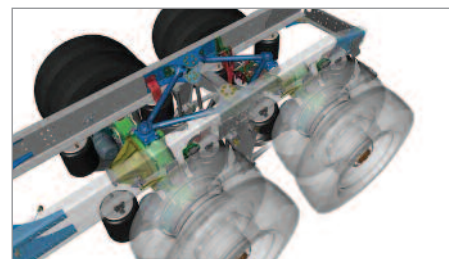
리어 에어서스펜션
