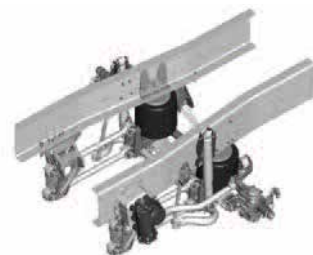
전축 에어서스펜션
