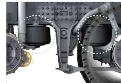
에어벨로우즈/스테빌라이저바
