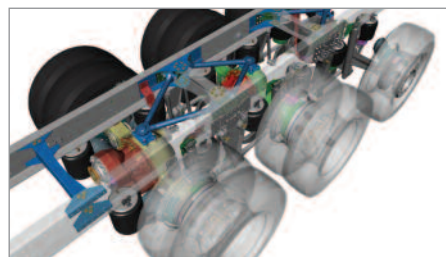
리어 에어서스펜션
