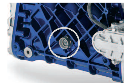
오일 레벨 점검창 점검창을 통해 오일을 점검할 수 있어 편리합니다.
