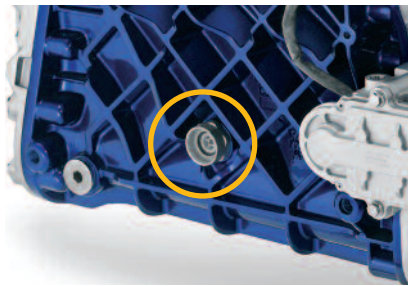
오일 레벨 점검창 점검창을 통해 오일을 점검할 수 있어 편리합니다.
