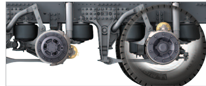
리어 에어서스펜션(FH 트라이덴)
