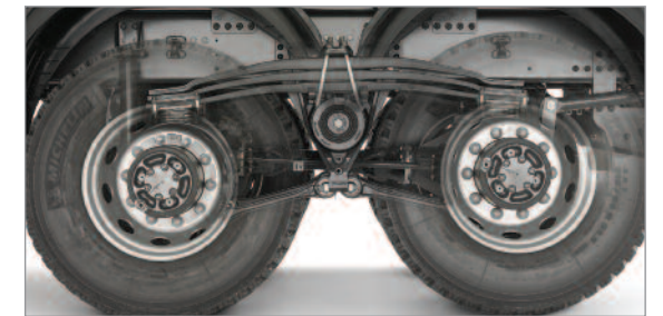
리어 리프서스펜션 (FM, FMX)
